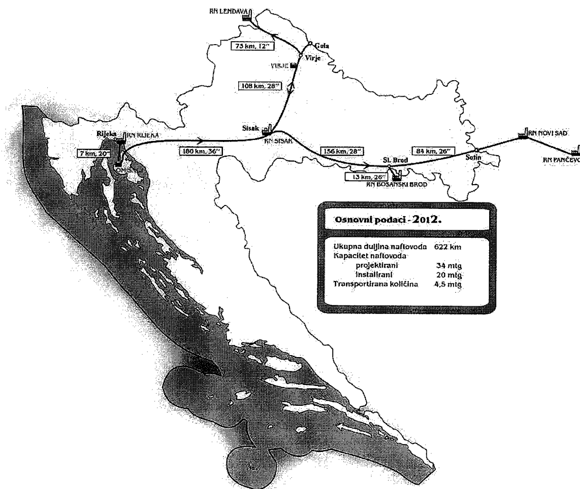
Slika 6.1.1. Naftovodni sustav JANAF-a d.d.
