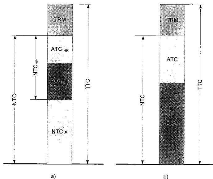
Slika 4.1.3. Načela određivanja prekograničnih prijenosnih kapaciteta
