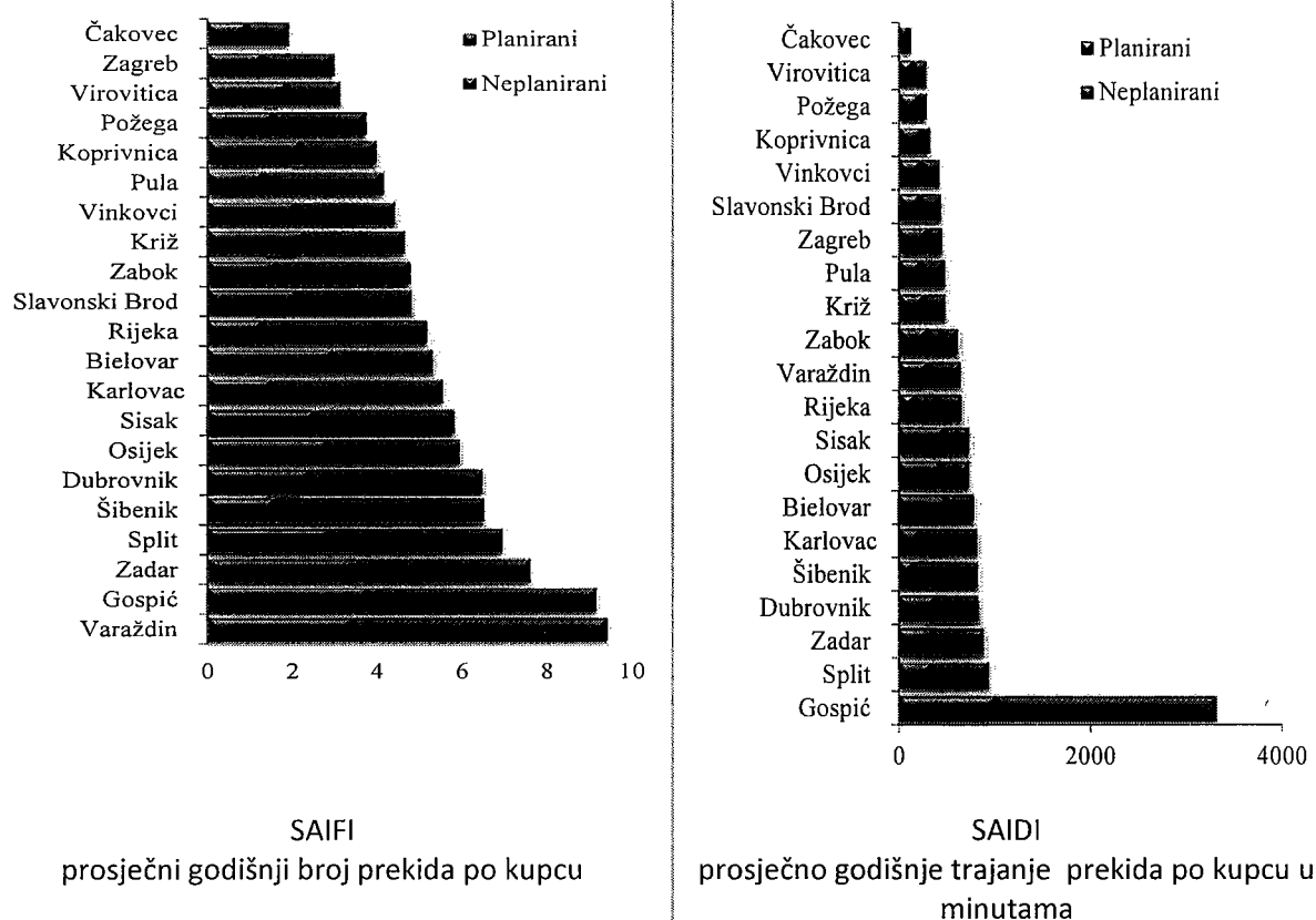
Slika 4.1.10. Pokazatelji pouzdanosti napajanja po distribucijskim područjima u 2012.
