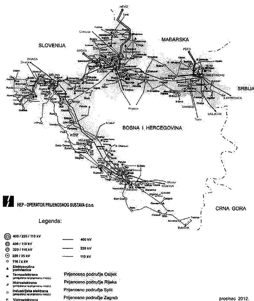
Slika 4.1.1. Shema prijenosne mreže i proizvodnih objekata hrvatskog elektroenergetskog sustava
