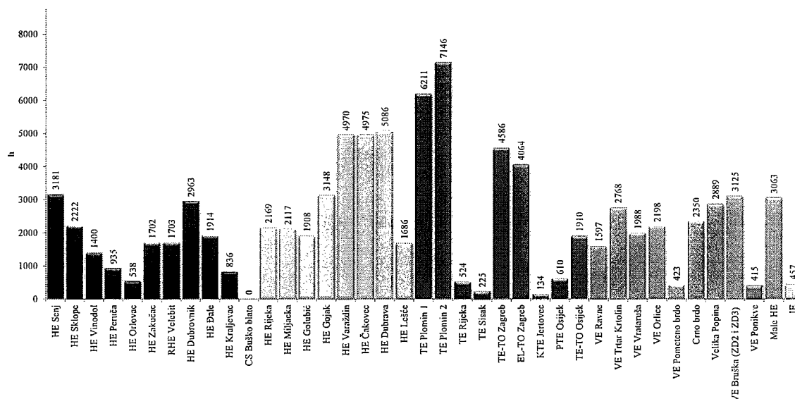
Slika 4.2.7. Trajanje vršnog opterećenja elektrana na teritoriju Republike Hrvatske u 2012.
