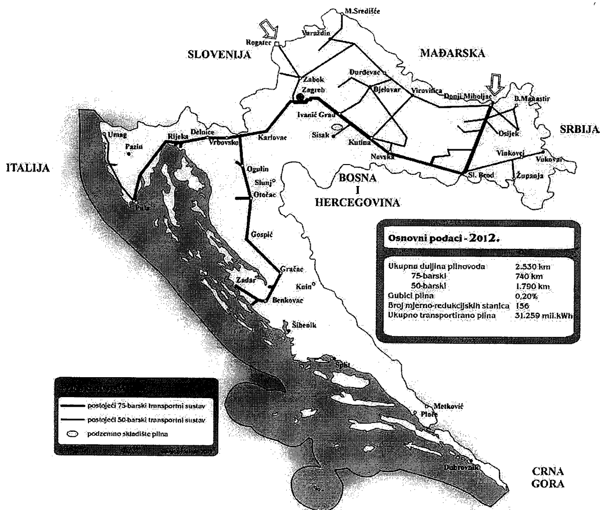
Slika 5.1.1. Postojeći plinski transportni sustav Republike Hrvatske
