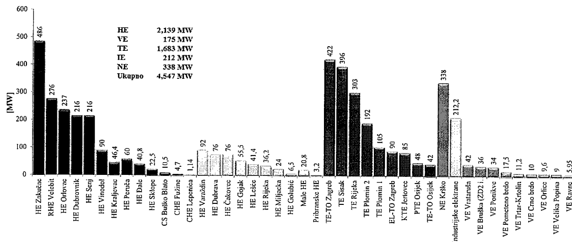
Slika 4.2.5. Raspoložive snage proizvodnih objekata u 2012.
