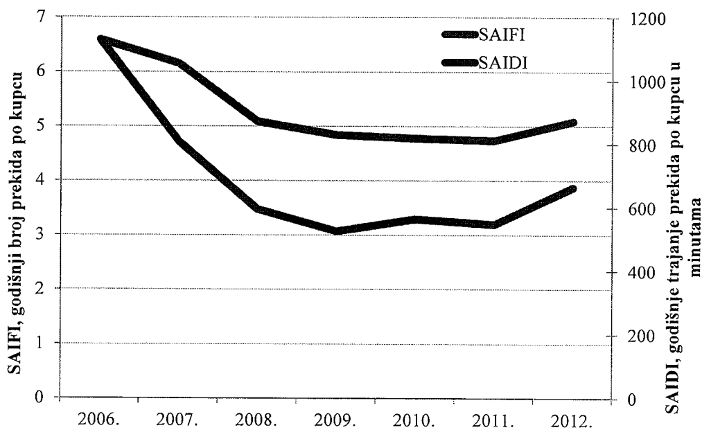
Slika 4.1.8. Pokazatelji pouzdanosti napajanja u HEP-ODS-u za 2012.
