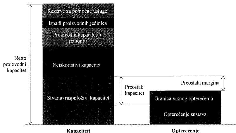
Slika 8.1.1. Načelo analize adekvatnosti proizvodnje
